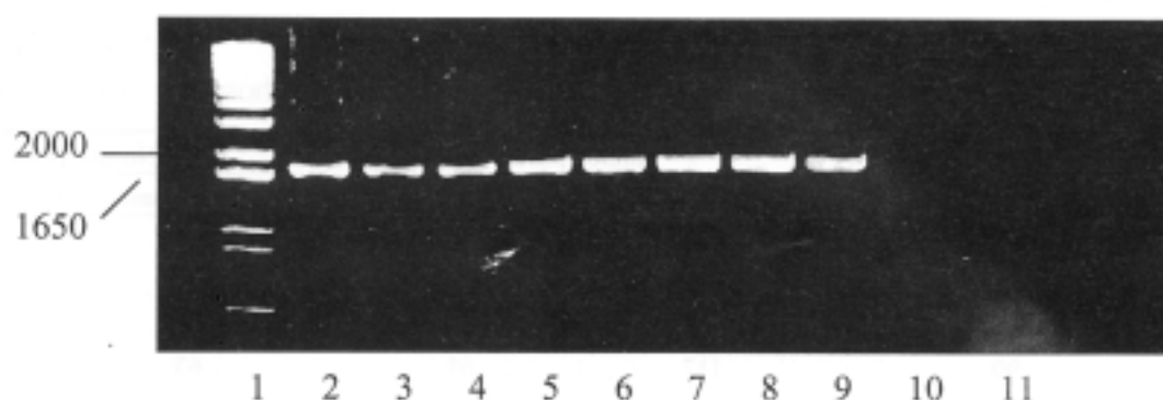
圖二 抗嘉磷塞轉基因大豆以 35S 及 NOS 為引子之 PCR 反應煉合溫度測定。第 1 欄為 DNA marker，第 2 欄至第 9 欄為分別為轉殖株之 PCR 煉合溫度 56、58、60、62、64、66、68、70 °C，第 10 欄為非轉殖株之 PCR 煉合溫度 56 °C，第 11 欄為去離子水
