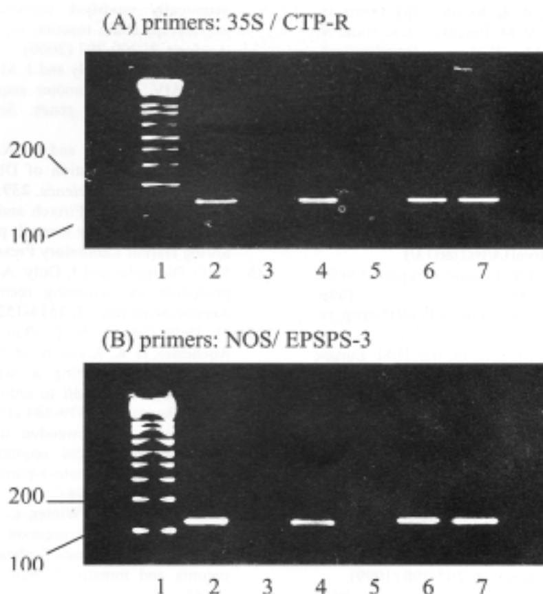
圖七 大豆及農產加工品抗嘉磷塞基因之 PCR 測定。純化之 DNA 以(A) 35S/CTP-R 及(B) NOS/EPSPS-3 為引子之增殖。第 1 欄為 DNA marker，第 2 欄為大豆葉片(轉殖株)，第 3 欄為大豆葉片(非轉殖株)，第 4 欄為大豆種子(0.1%、轉殖株/非轉殖株)，第 5 欄為大豆種子(非轉殖株)，第 6 欄為豆漿，第 7 欄為豆腐
